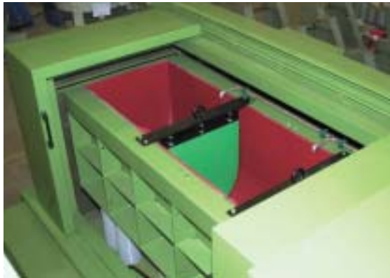
Vályú hangszigetelő fülkével
